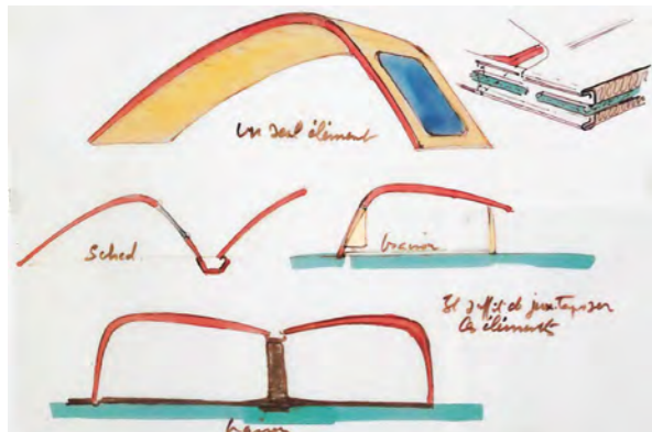
Le Pavillon du centenaire de l'aluminium, 1954
