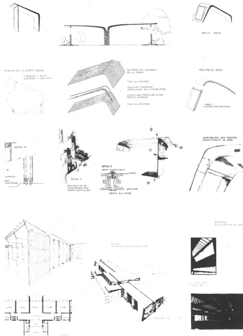
Analyse des systèmes constructifs, coque et voûte, 1976
